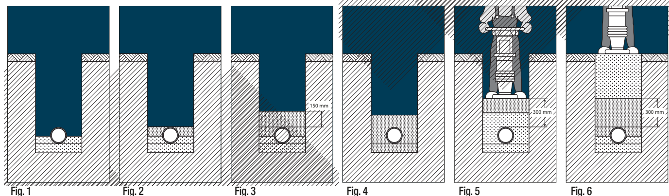
Fig. 1 – Strato di materiale di riempimento compattato a mano
